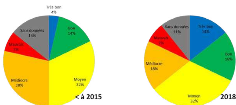
Figure 14 : Evolution des évaluations sur les éléments de qualité nutriments, phytoplancton et macrophytes entre les deux SDAGE (2016-2021 et 2022-2027)
