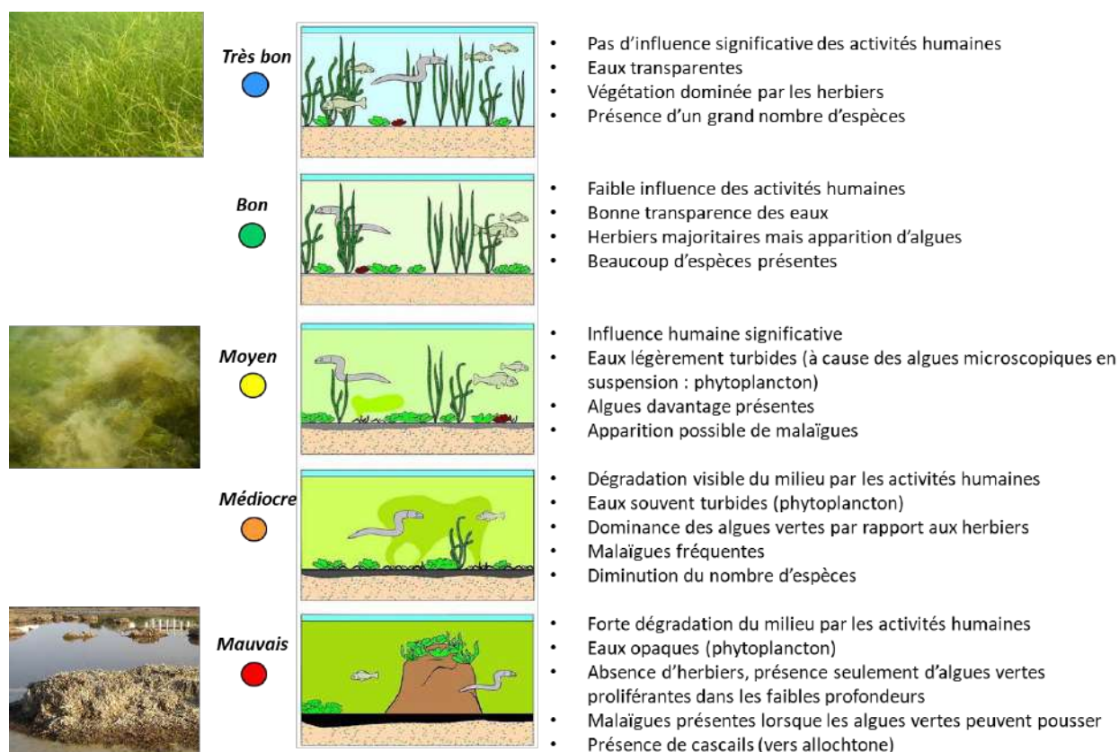
Figure 2 : Illustration des niveaux d'eutrophisation dans les lagunes
