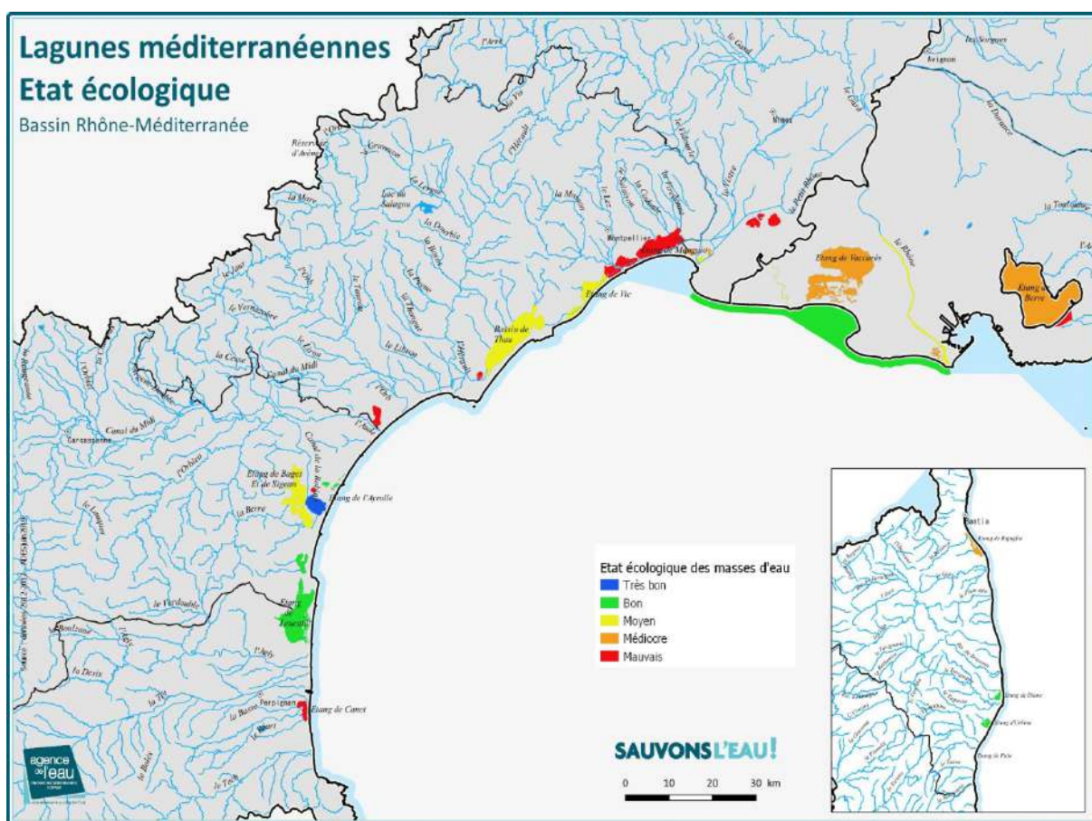
Figure 11 : Carte de l'état écologique des masses d'eau lagunaires en 2018
