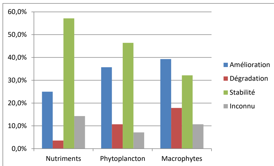
Figure 13 : Evolution des masses d'eau (en pourcentage) sur les compartiments nutriments, phytoplancton et macrophytes entre les deux états des lieux des SDAGE 2016-2021 et 2022-2027
