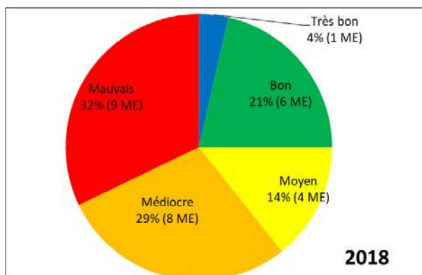
Figure 10 : Etat écologique des masses d'eau lagunaires de Rhône-Méditerranée et de Corse en 2018
