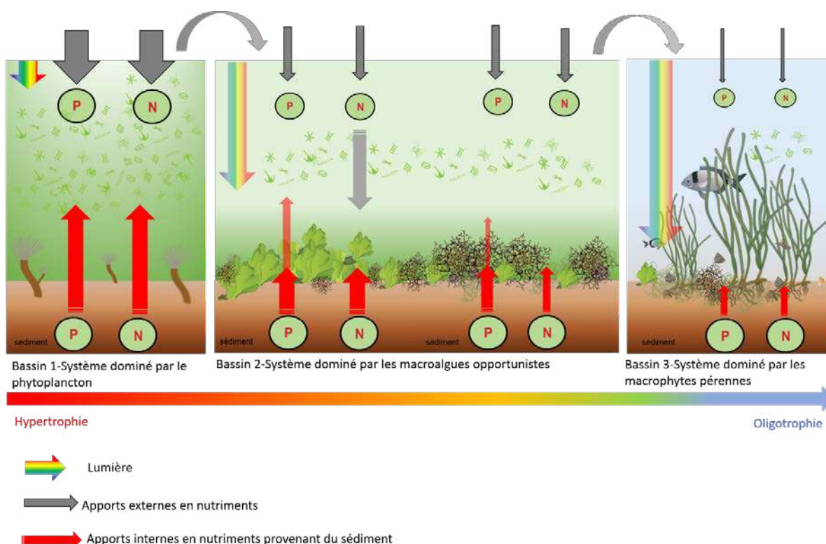
Figure 15 : Représentation de l'impact de la réduction des apports en nutriments sur le changement au sein des producteurs primaires et du rôle des communautés sur les flux d'azote et de phosphore (Le Fur, 2018)
