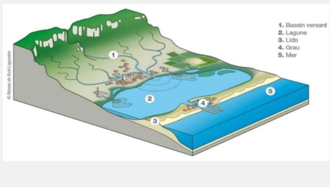
Figure 1 : Schéma d'une lagune (source : Réseau de Suivi Lagunaire)
