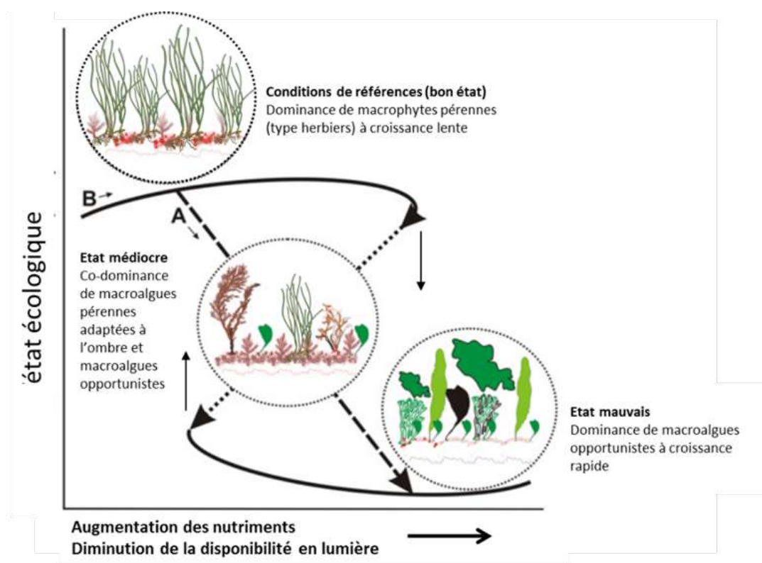
Figure 5 : Modèle conceptuel de deux états stables alternatifs des macrophytes marines benthiques selon le gradient d'eutrophisation dans les lagunes. (A) changement de la végétation continue et graduelle en réponse à l'augmentation des nutriments (B) changement discontinu : l'état du système varie peu jusqu'à l'atteinte d'une valeur seuil ; l'écosystème bascule vers un autre état et un autre mode de fonctionnement (Le Fur, 2018).
