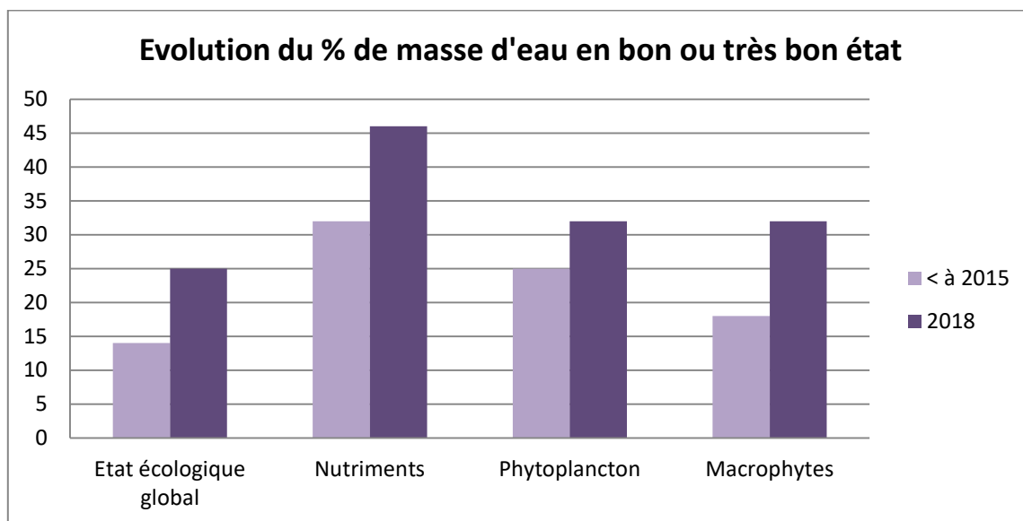
Figure 12 : Evolution du pourcentage de masse d'eau en bon ou très bon état entre les deux états des lieux des SDAGE 2016-2021 et 2022-2027
